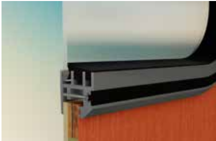
Montage mit innerer Gegenleiste (Standard - OMRU TL)
