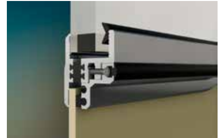
Montage mit innerer Gegenleiste (thermisch getrennt - OMRU THERMO)
