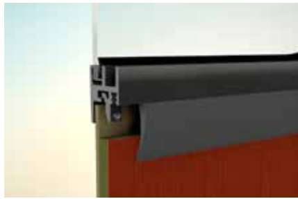
Montage mit Klemmblocken (Standard)
