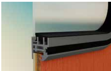
Montage d.m.v. tegenlijst binnenzijde (standaard)
