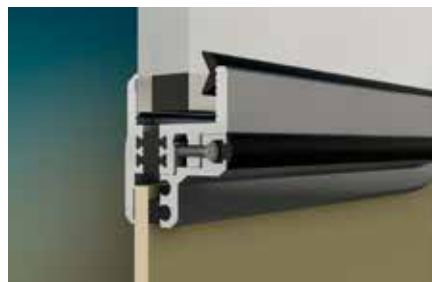
Montage d.m.v. tegenlijst binnenzijde (thermisch onderbroken)
